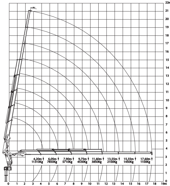
Gráfico de Carga | Gráfico de carga
