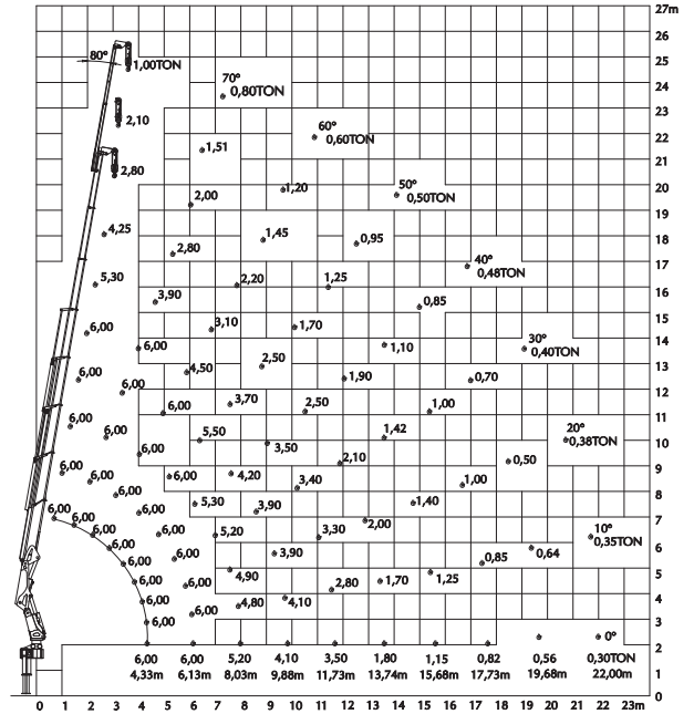
Gráfico de Carga com Guincho e lança JIB | Gráfico de Carga com Guinche y Plumín
